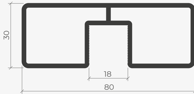
80x30x18mm Üst Küpeşte
