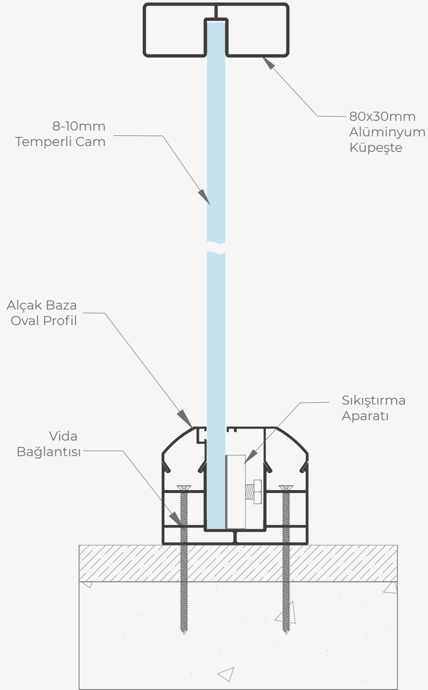
Alçak Baza Bağlantı Detayı
