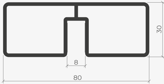
80x30x8mm Üst Küpeşte
