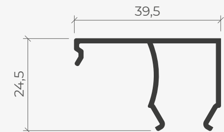
Düz Çıta (Kulaklı)
