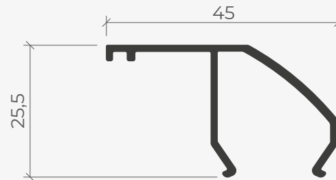
Oval Çıta (Kulaklı)
