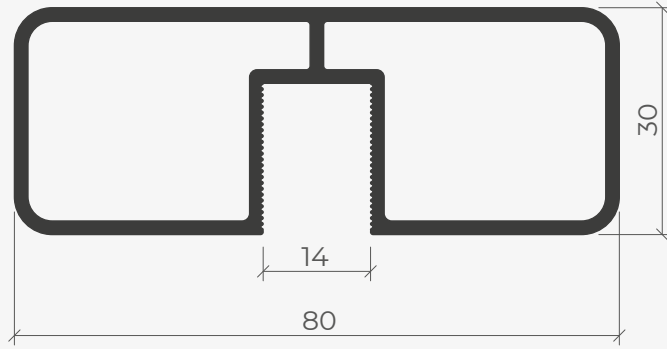
80x30x14mm Üst Küpeşte
