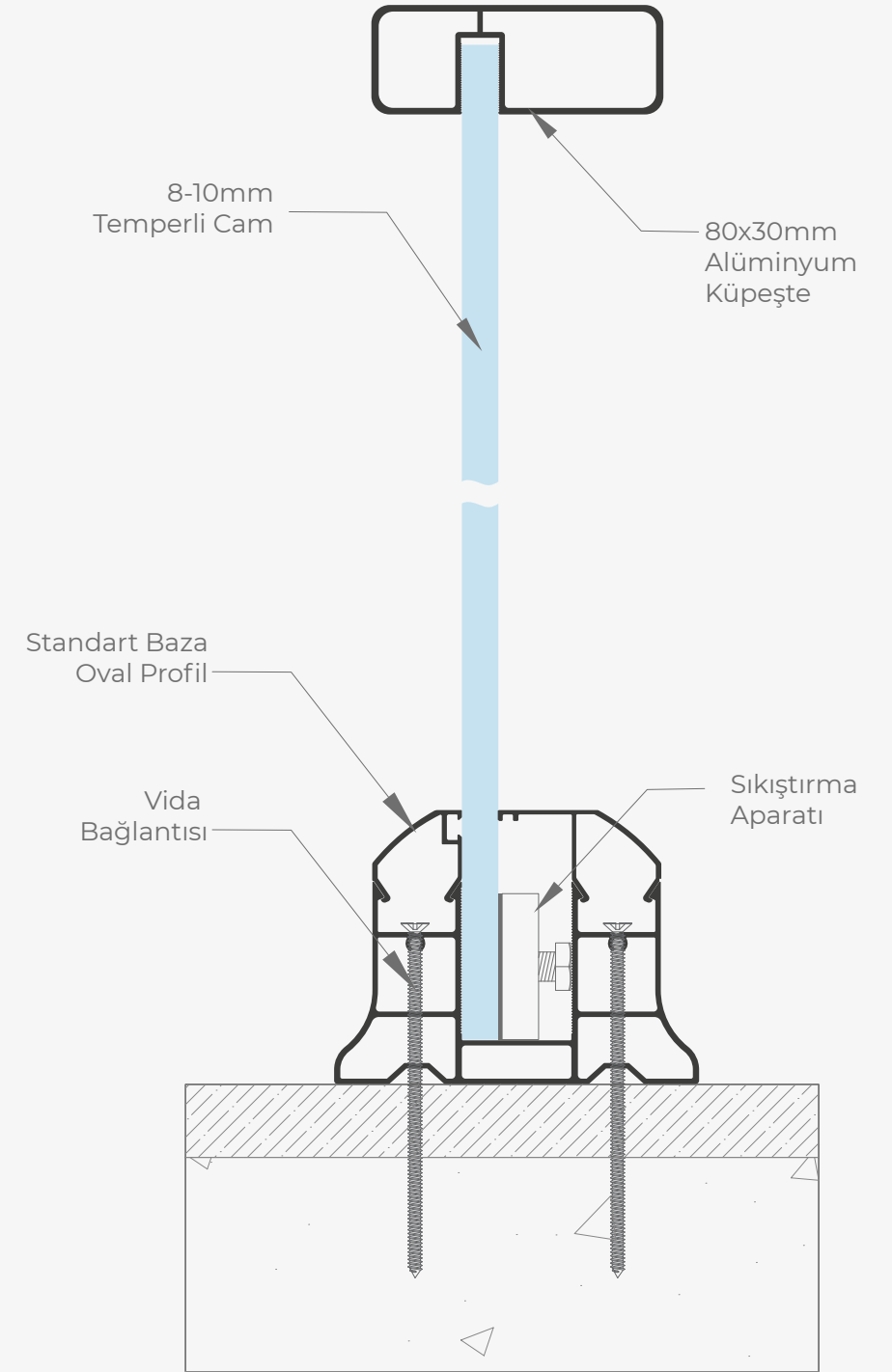
Standart Baza Bağlantı Detayı
