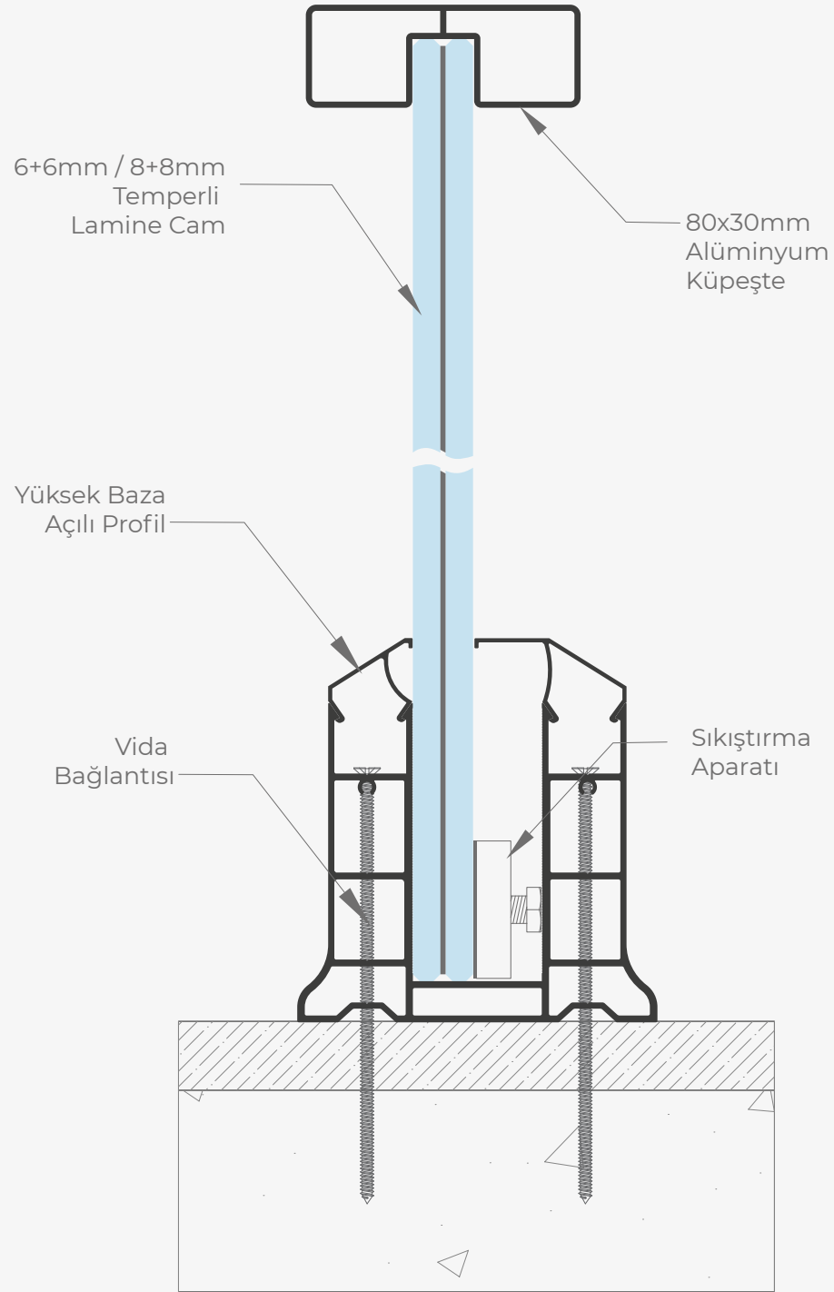
Yüksek Baza Bağlantı Detayı
