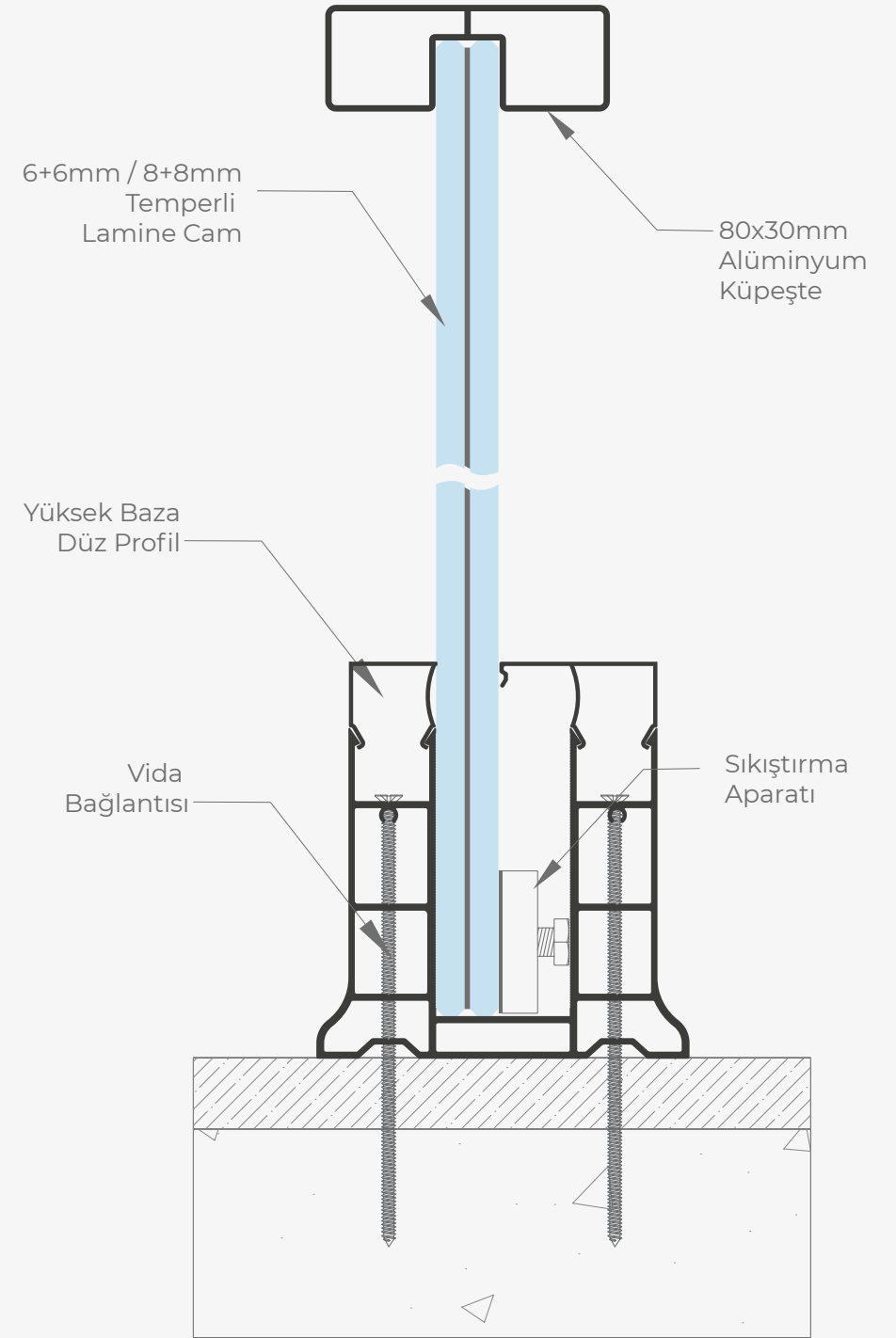
Yüksek Baza Bağlantı Detayı (Düz Çita Kullanımı)
