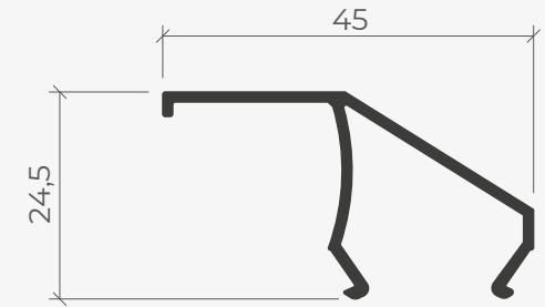
Açılı Çıta (Kulaklı)
